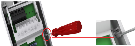
Rys 3 – Wyjmowanie modułu elektronicznego
